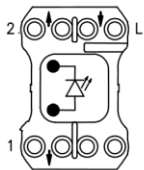
Łącznik schodowy 10A Two-way switch 10A
